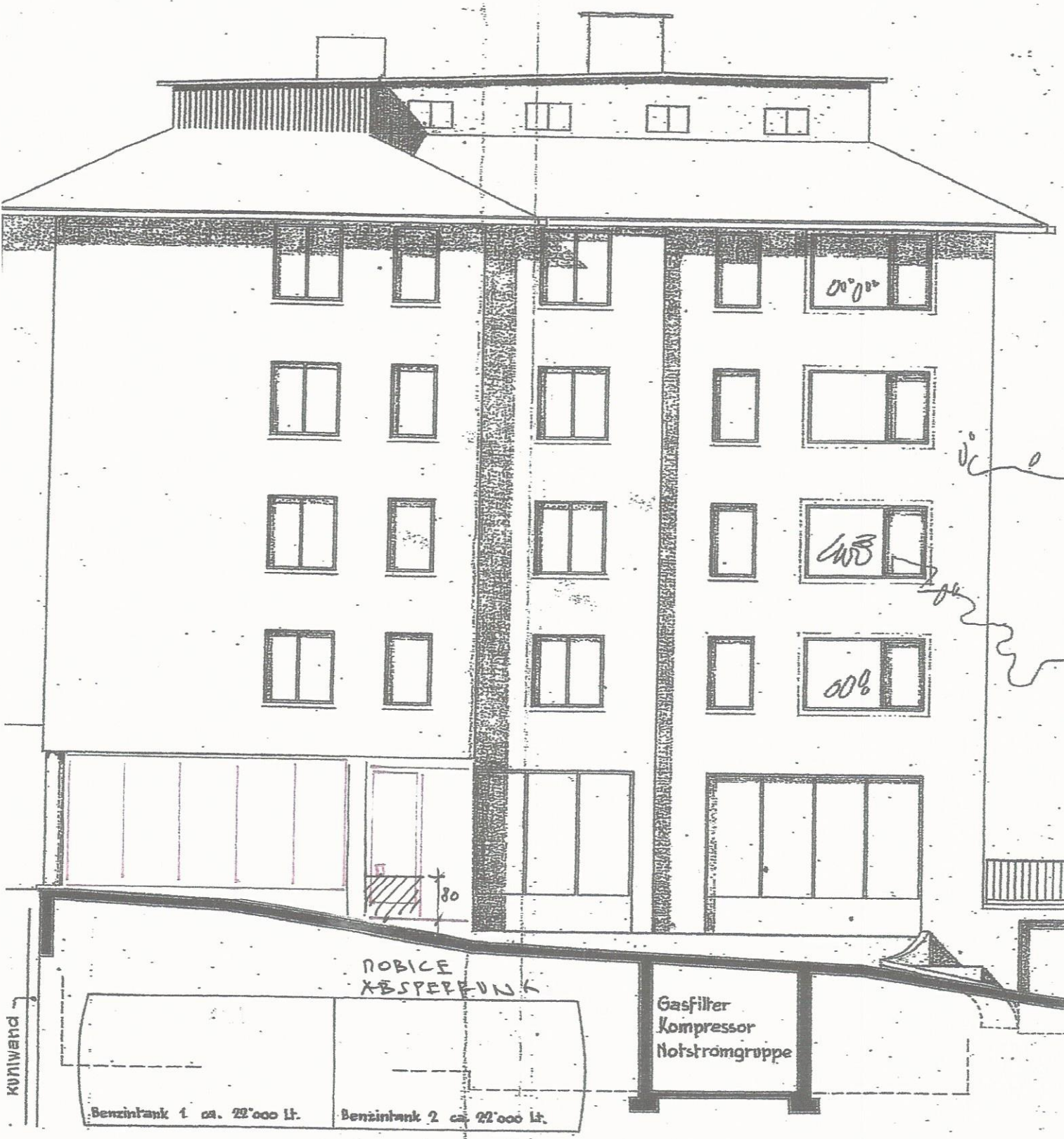
SÜDOST — ANSICHT
